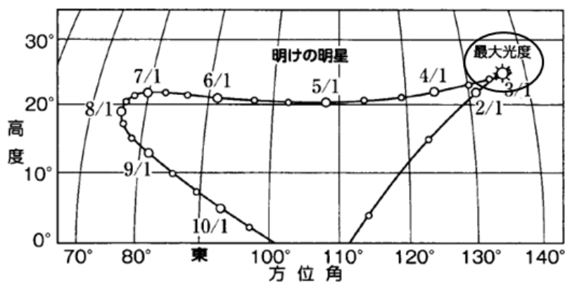
日出時の金星の高度と方位角(東京での値)
