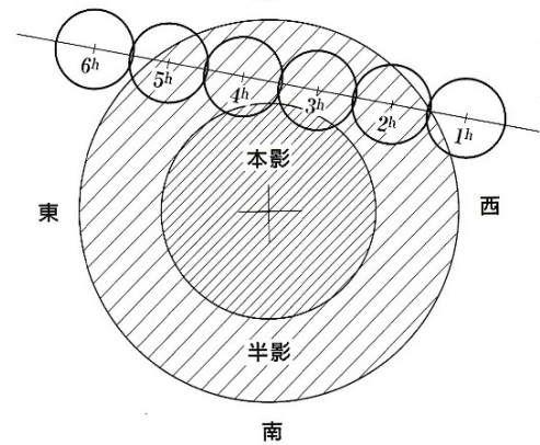
図7 8月8日の部分月食
