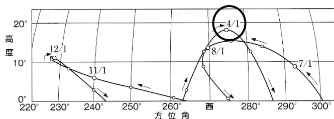
図3 日没時の水星の高度と方位角 (東京での値)
